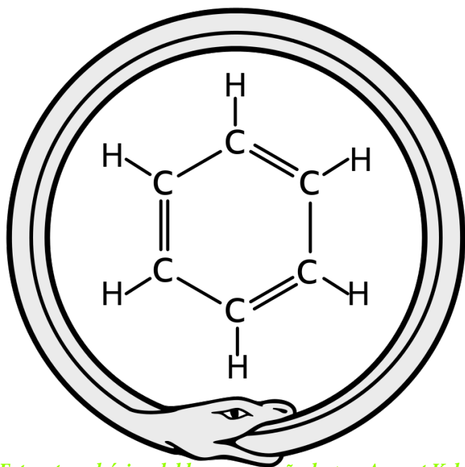
Estructura básica del benceno, soñada por August Kekulé en 1865
